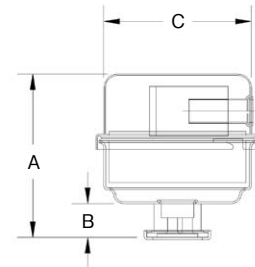
真空ポンプの排気側に取り付けた EFS排気フィルタサイレンサの例
