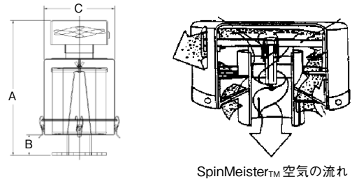
SpinMeister™ 空気の流れ
